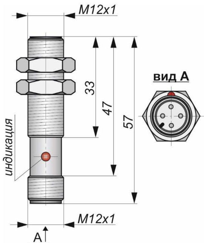
Габаритный чертеж
